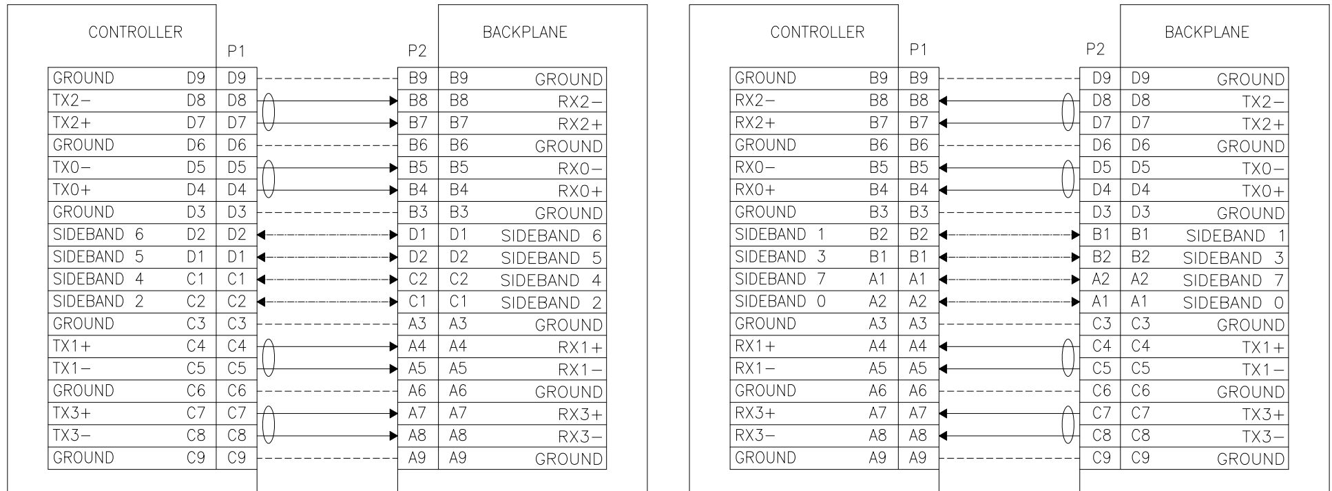
WIRING TABLE
